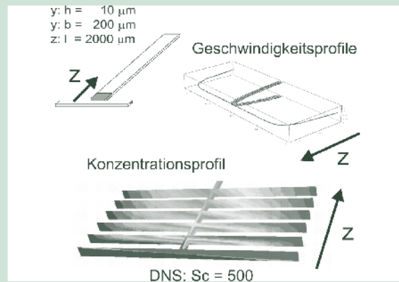
Flachbettmikroreaktor: Modellbasierte Messung und Auswertung
