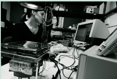
Photovoltaik-Messplatz
