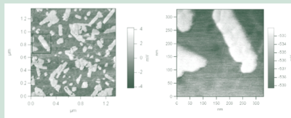
Reibungs-Kraft Analyse von Nanoclays auf Gold
