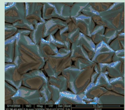
REM-Aufnahme von Sb-Kristalliten
