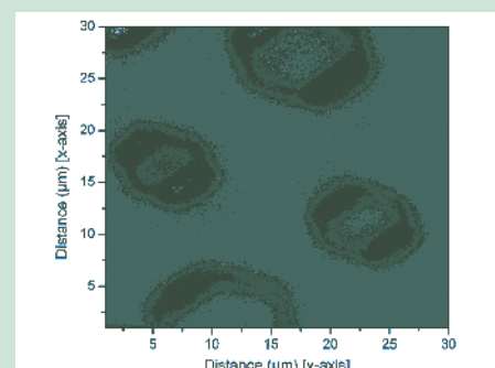
Nichtlineare Mikroskopie an ferroelektrischen Domänen in Lithiumniobat
