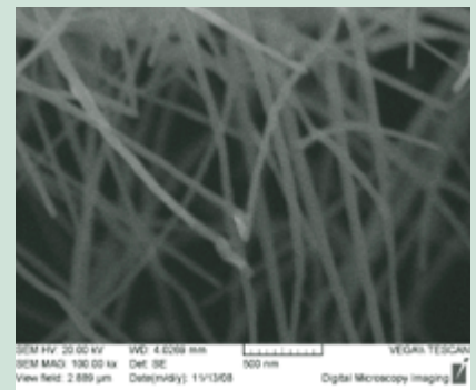
REM-Aufnahme von Bi-Nanowires
