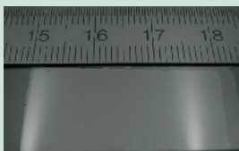
\text{LiNbO}_3 auf \text{SiO}_2 auf \text{LiNbO}_3
